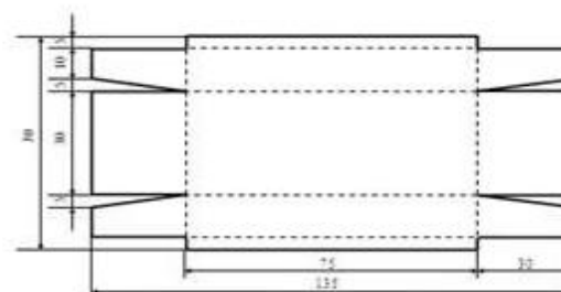
Шаблон развёртки изделия «Кормушка для птиц»
